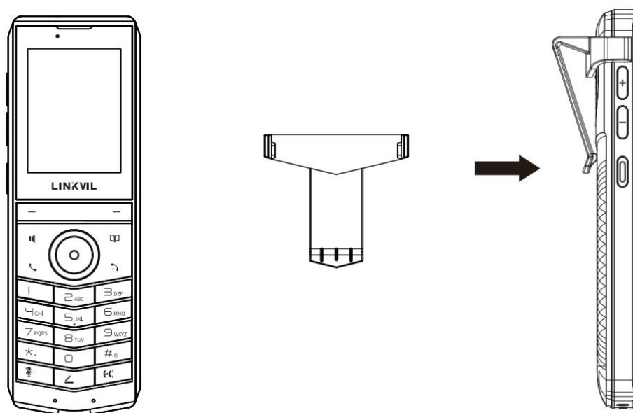
图 5 - 安装腰带夹
